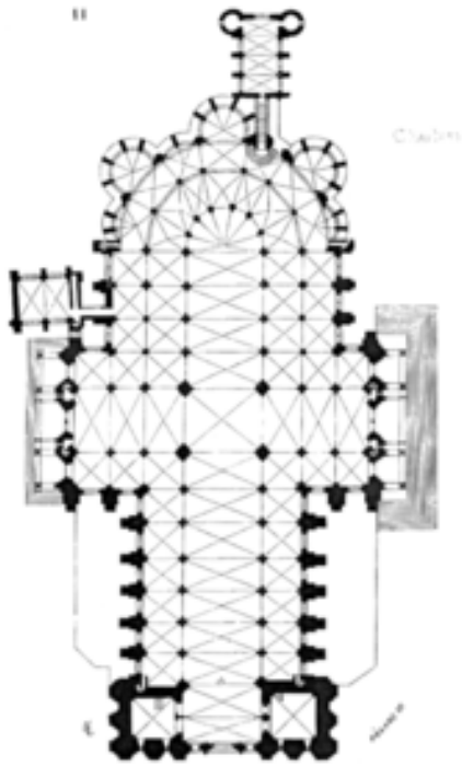
Planta de la catedral de Chartres (Francia)
